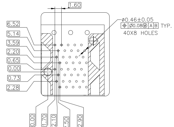
DETAIL H 2:1
