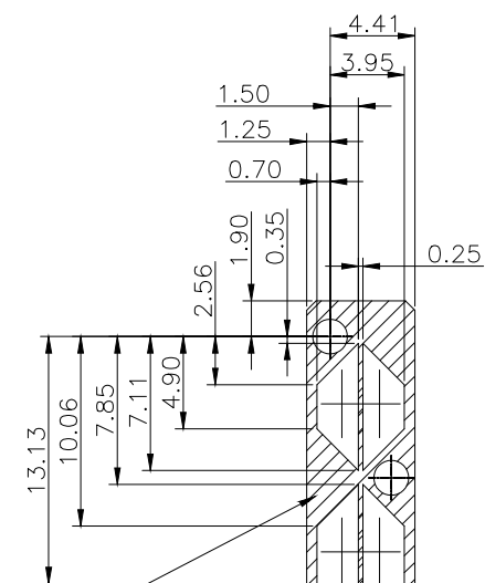
DETAIL H 2:1
