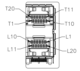
DETAIL A 1:1
